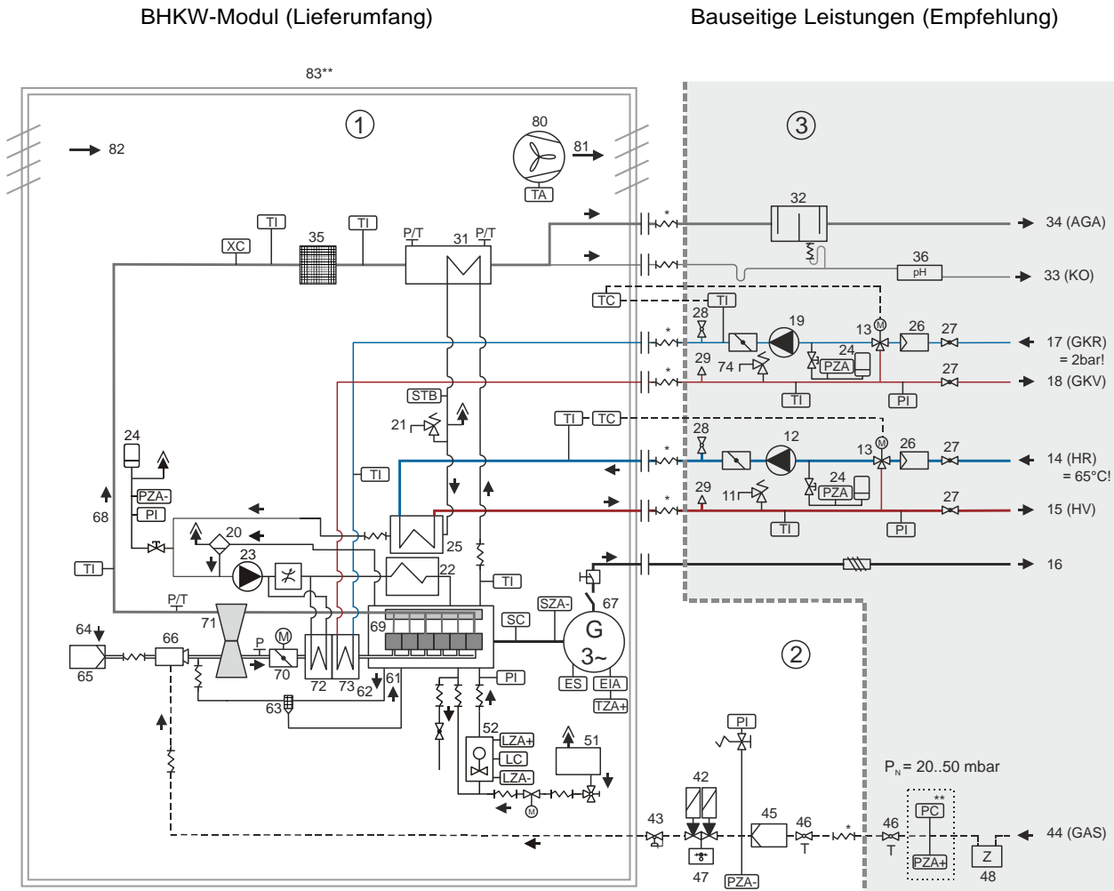
Abb. 2 Überwachungseinrichtungen Variante Vitobloc 200 EM-199/263 mit separatem Niedertemperaturkreis; (Pos. 80 und 83 optional) Wenn der Systemdruck in dem Gemisch-Kühlwasserkreis (17+18) über 2 bar liegt, ist kundenseitig eine hydraulische Trennung vorzusehen!
