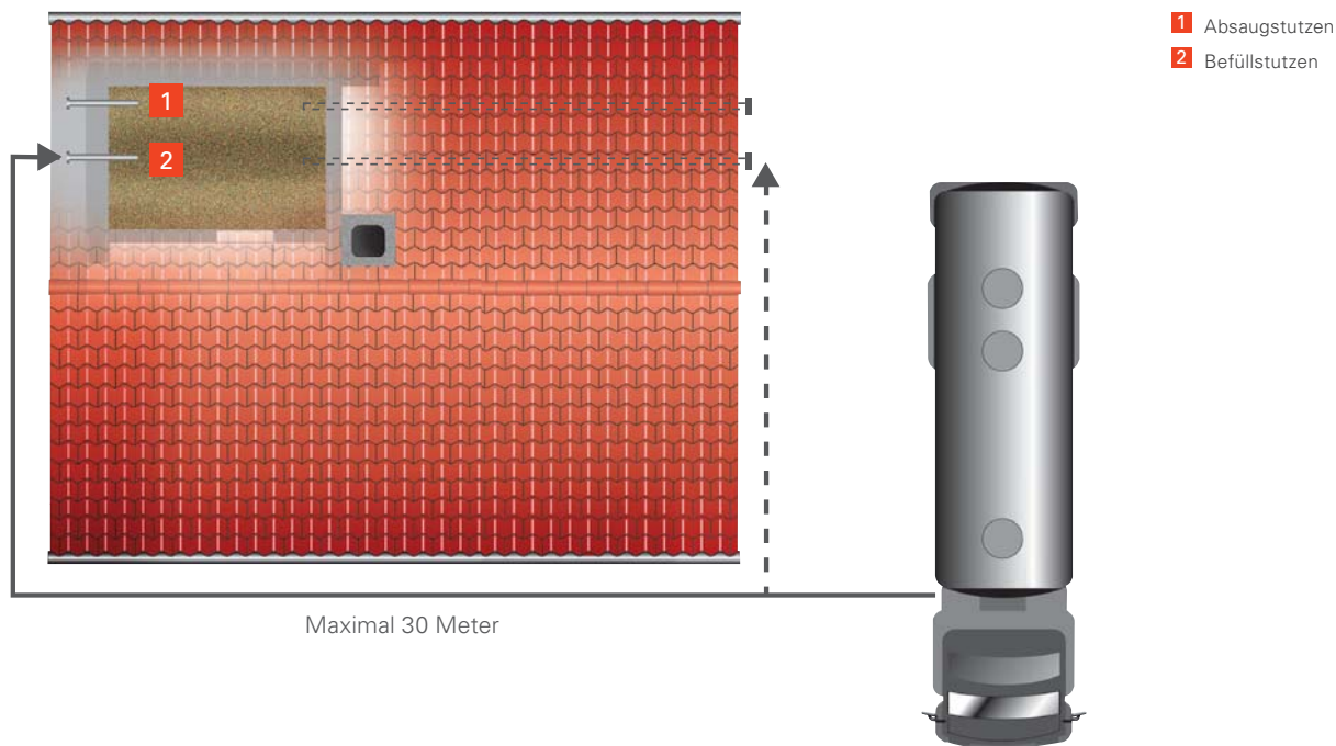
Lage des Pelletlagerraums
