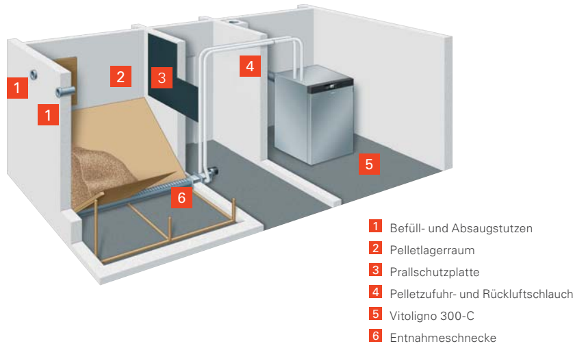
Einbaubeispiel Lagerraum mit Zuführung zum Pelletkessel durch Vakuum-Saugsystem
