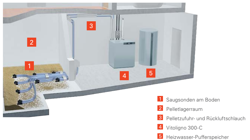
Lagerraum ohne Schrägboden mit Zuführung zum Pelletkessel über Saugsonden
